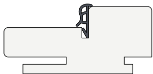
Коробка «Т» 2070×70×32
